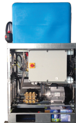
TELAIO POMPE
